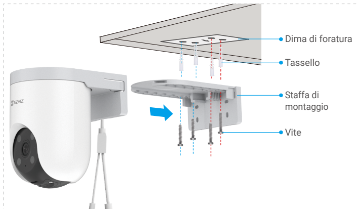
Fig. 1 Montaggio a soffitto
